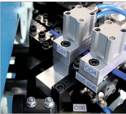
Unidad de alimentación de banda y cizalla.
